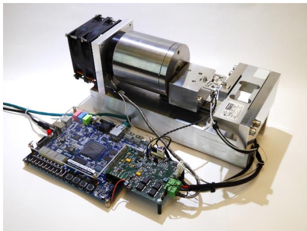
Bild 2: Prüfstand mit Aktor und Referenzsensor sowie der Auswerteschaltung
