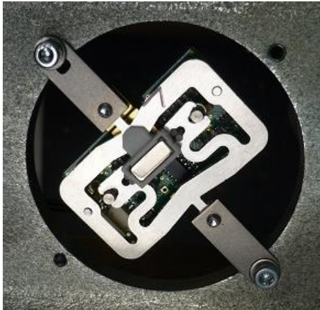
Bild 1: Wägezelle der Firma Digisens
